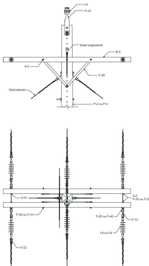
Figura 67 – Estrutura TE – Poste de seção DT ou de madeira
