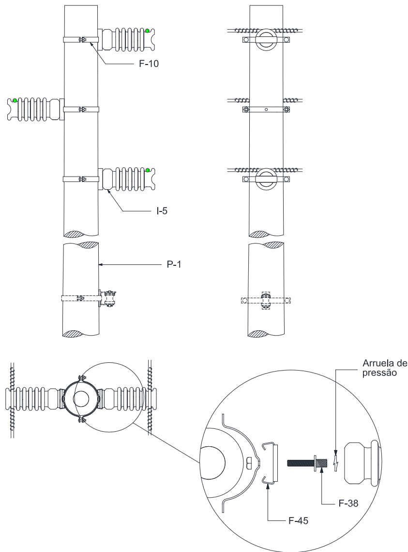
Figura 76 – Estrutura P1 – Poste de Seção Circular
