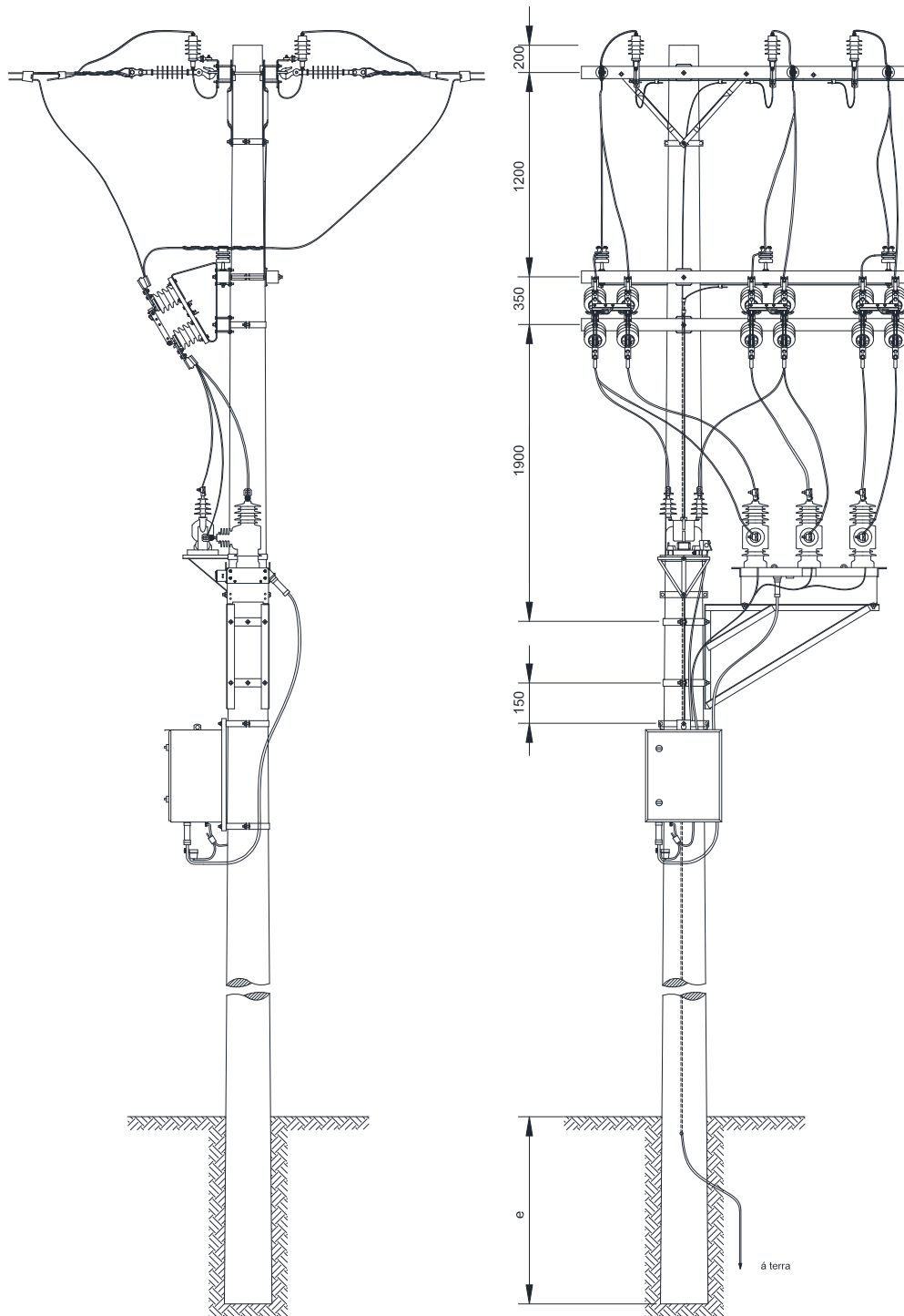
Figura 132 – Instalação de equipamento – Religador – Seccionamento tipo faca “bay-pass” – Para-raios no 1º nível
